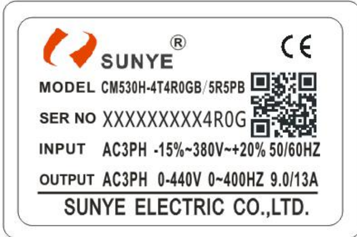
图2-2. 铭牌
