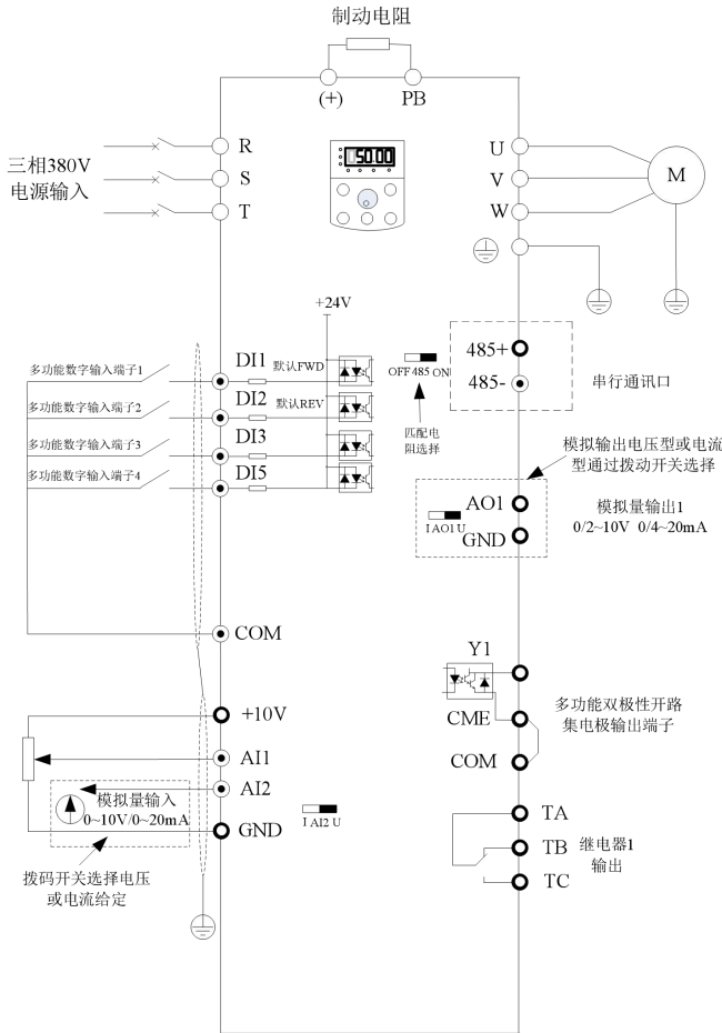
图 3-1. 1.5kW 以下三相变频器
