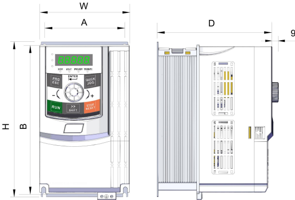
图 2-3. 15KW 以下塑胶外形尺寸及安装尺寸示意图
