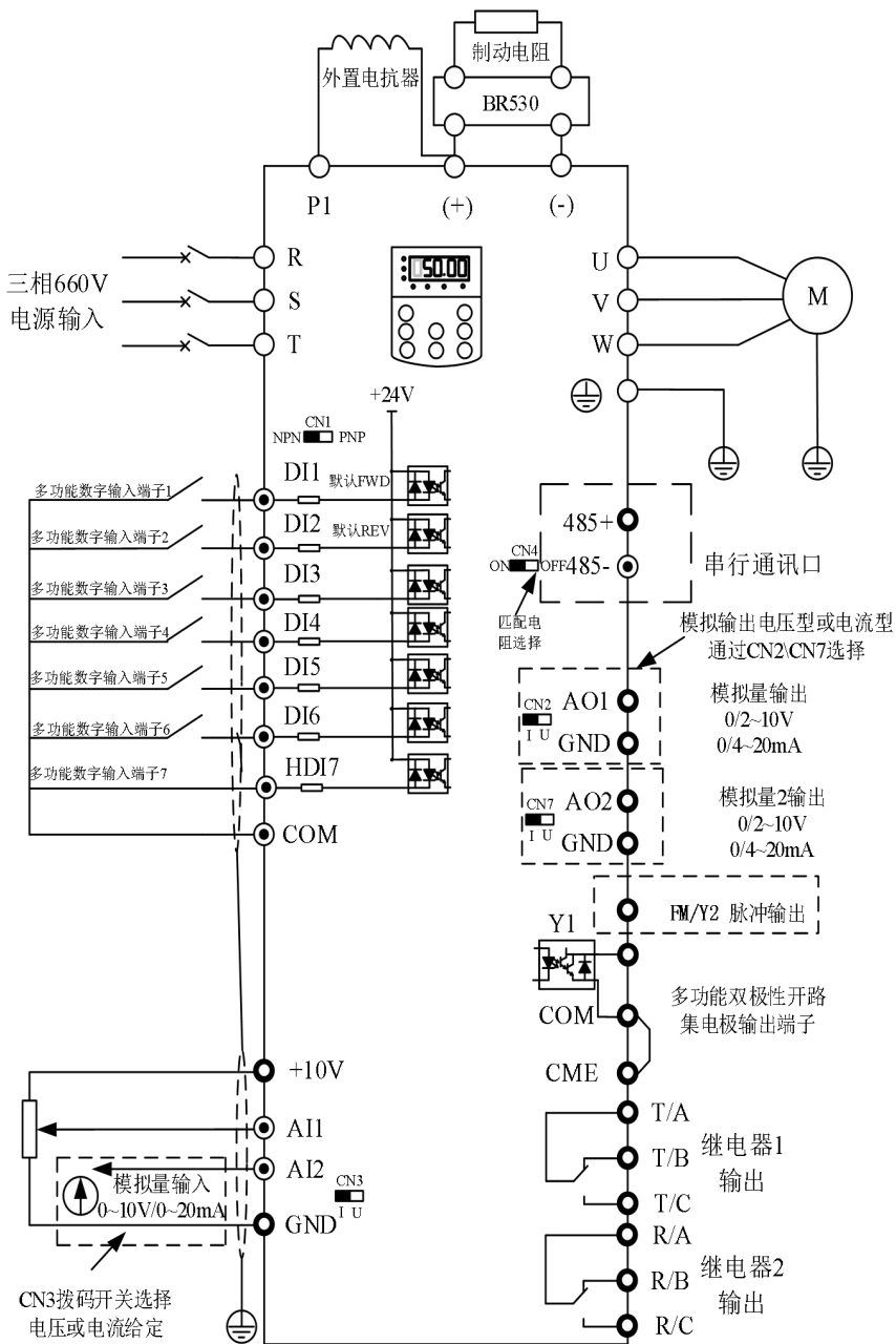
图 3-10. (7T) 75Kw 及以上三相变频器
