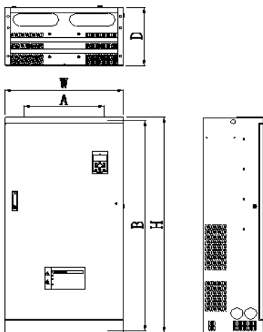
图 2-6. 160KW 以上变频器外型尺寸及安装尺寸示意图
