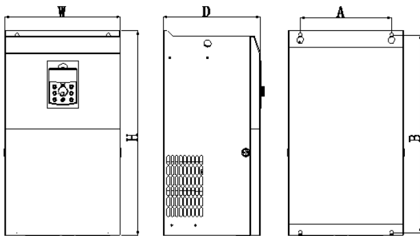
图 2-5. 45~132KW 变频器外型尺寸及安装尺寸示意图
