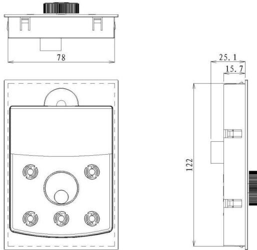
图2-7. 外引键盘带托盘安装尺寸图
