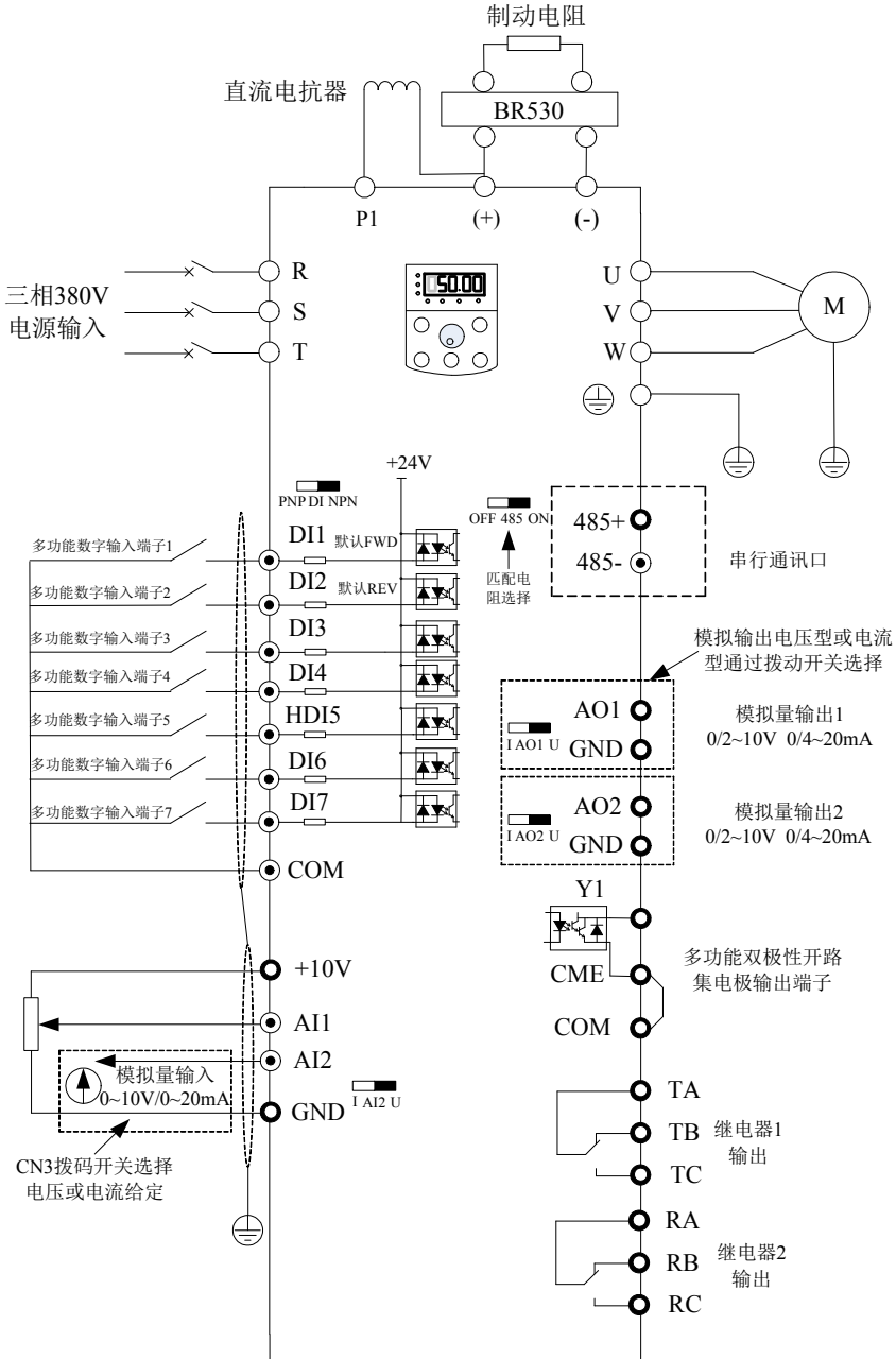
图 3-4. (4T) 75Kw 及以上三相变频器
