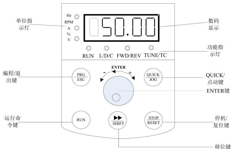
操作面板示意图1(标准配置LED键盘1)
