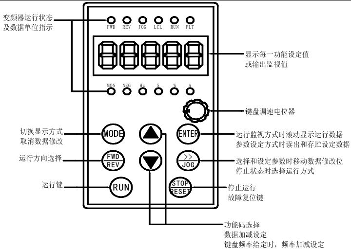
图4-1. (7T-75KW以上系列) 操作面板示意图(标准配置LED键盘)
