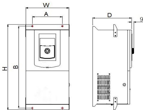
图 2-4. 18.5~37KW 钣金机箱外形尺寸及安装尺寸示意图
