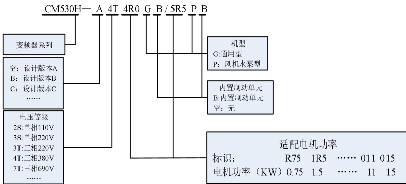
图2-1. 命名规格
