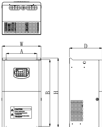
图 2-4. 22~132KW 变频器外型尺寸及安装尺寸示意图
